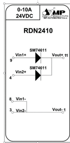
Slika 1. Principijelna šema modula RDN 2410 sa ulazno-izlaznim priključcima (modul za napone do 26VDC)
