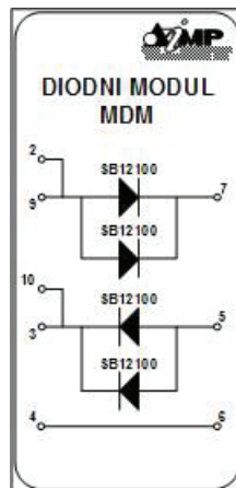
Slika 1. Principijelna šema modula MDM sa ulazno-izlaznim priključcima (modul za napone do 100Vdc)
